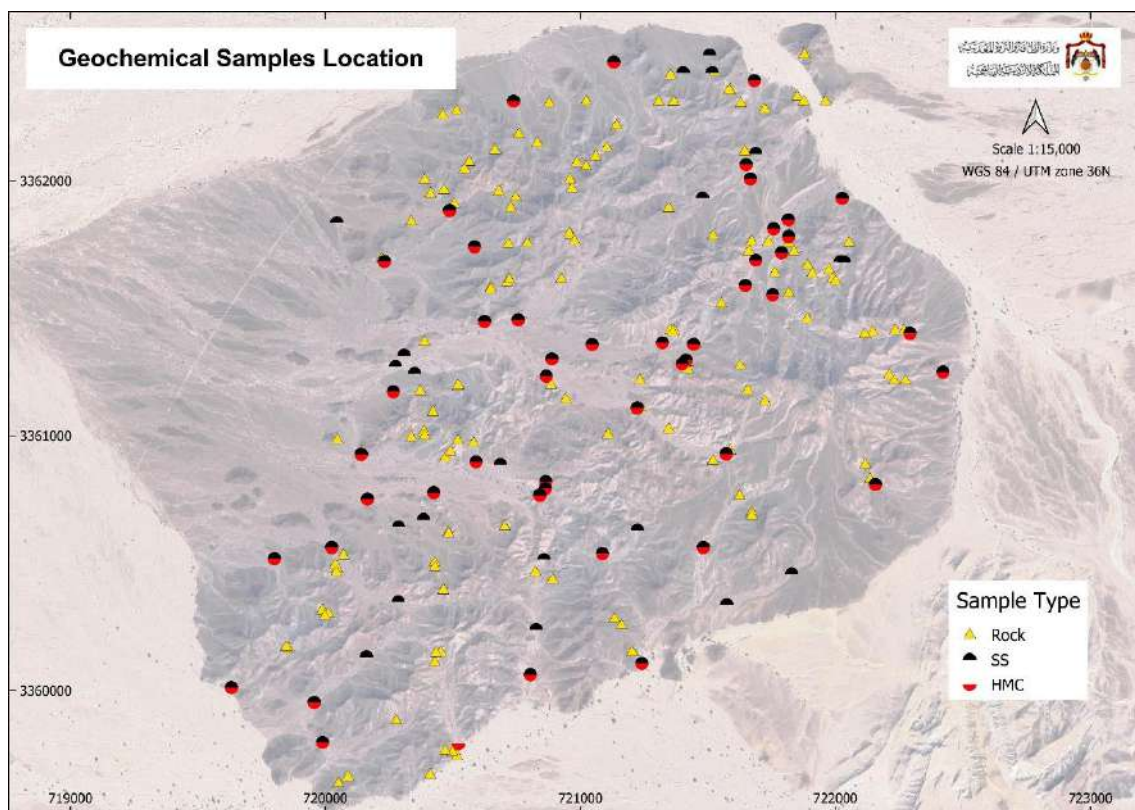
شكل 11: مواقع العينات الجيوكيميائية في منطقة الدراسة.
