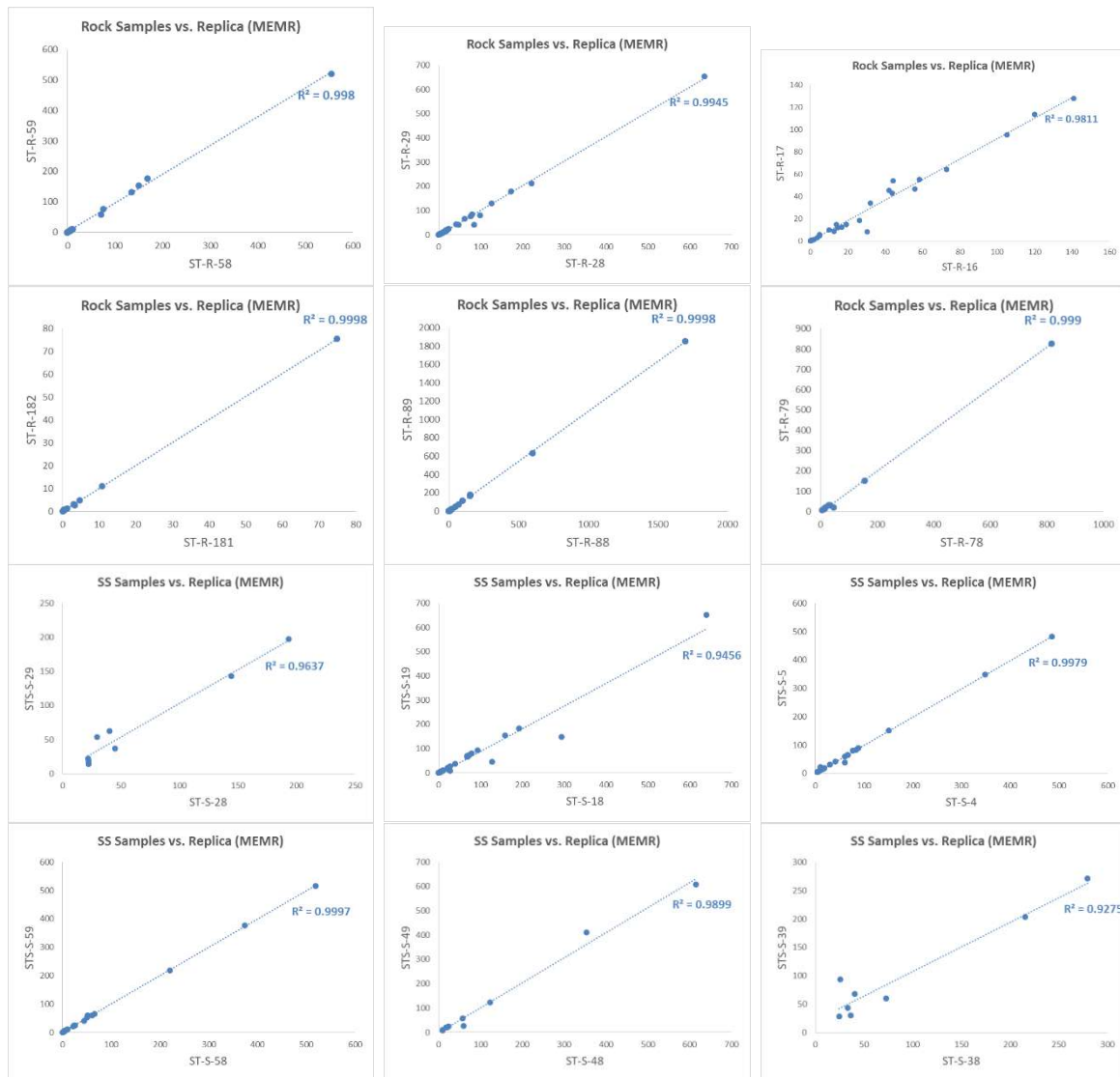
شكل 16: مدى المقاربة في عينات الرقابة الصخرية ولرسوبيات الأودية.
